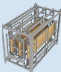
Art. Nr. 34400 elea Transportgerüst für 3 Stk. Betonierbühne 2000 für Hohlwände
